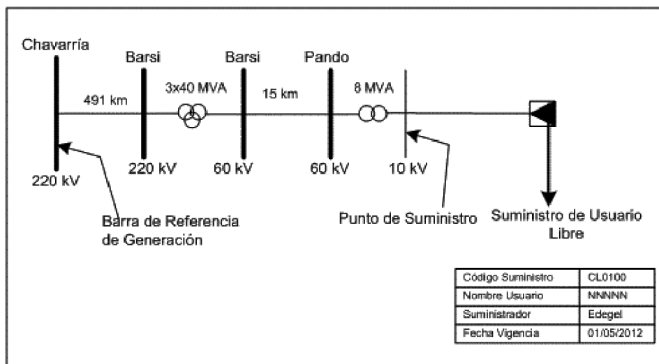
FIGURA 1 Diagrama Unifilar del Suministro del Usuario Libre
